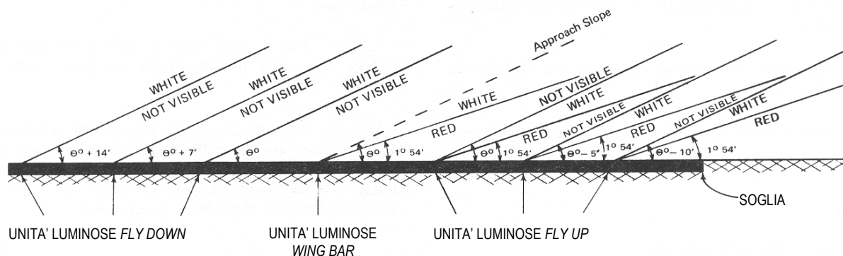
Figura 6.10 – Angoli di regolazione delle unità T-VASIS e AT-VASIS
