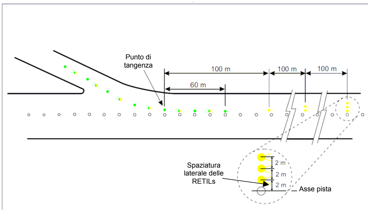
Figura 6 – 16B - Luci di segnalazione di raccordo d'uscita rapida (RETILs)
