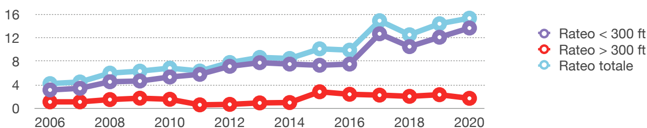
Trend nazionale dell'indice di rischio medio annuale (n. impatti/10.000 movimenti) per aviazione commerciale (2006-2020)
