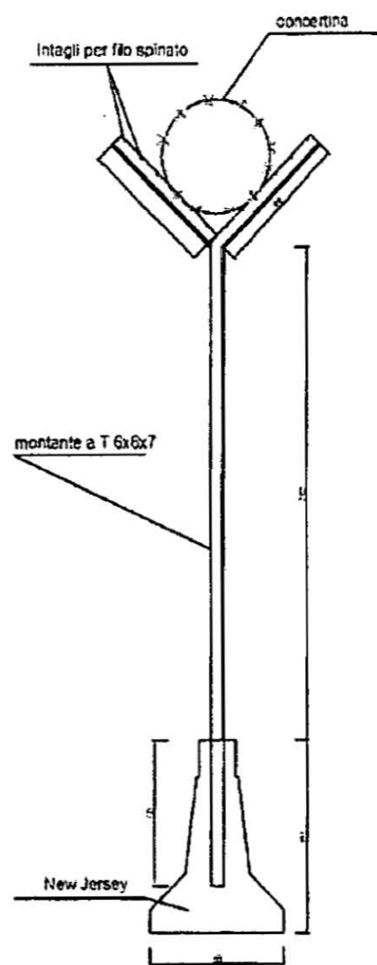
Figura 1: Schema recinzione doganale provvisoria
