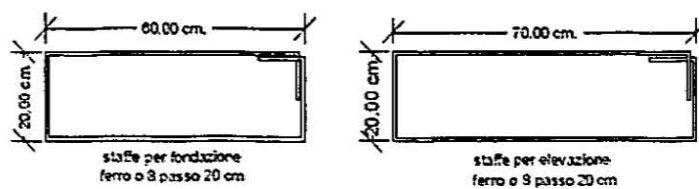
PARTICOLARI STAFFE PER ARMATURA MURO
