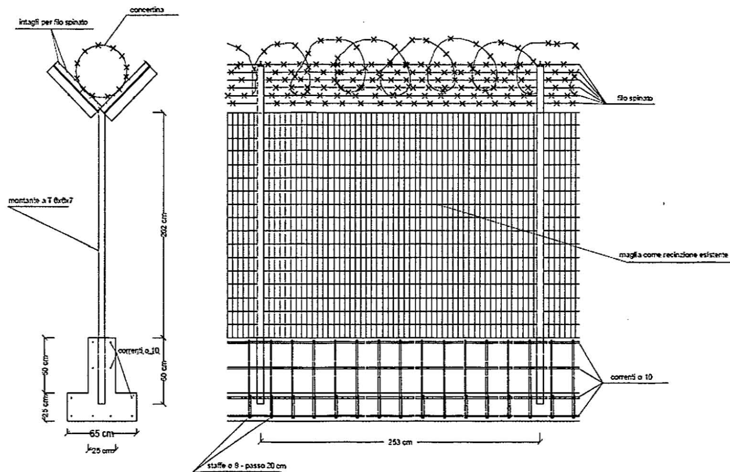
Figura 2: Schema nuova recinzione doganale
